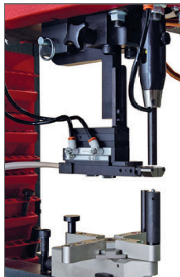
螺母、螺钉和螺柱在 Multi-Shuttle 工具平台的使用
