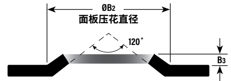
压花安装孔 (1)
