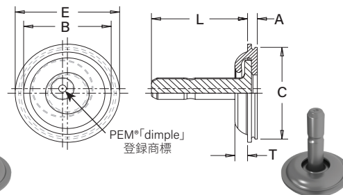
MRHPS グループ付きピン
