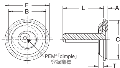
MRPS スムースピン
