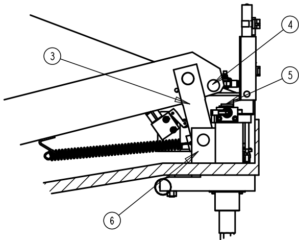
Préskulissza oldalnézetben
