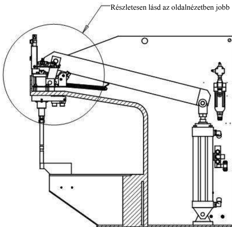
Présgép szerkezeti felépítése Ábra 3.2-2
