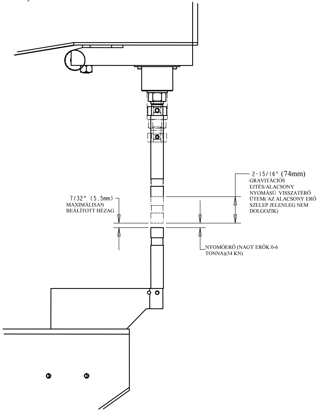
LÖKETHOSSZ ÁBRA 4.0
