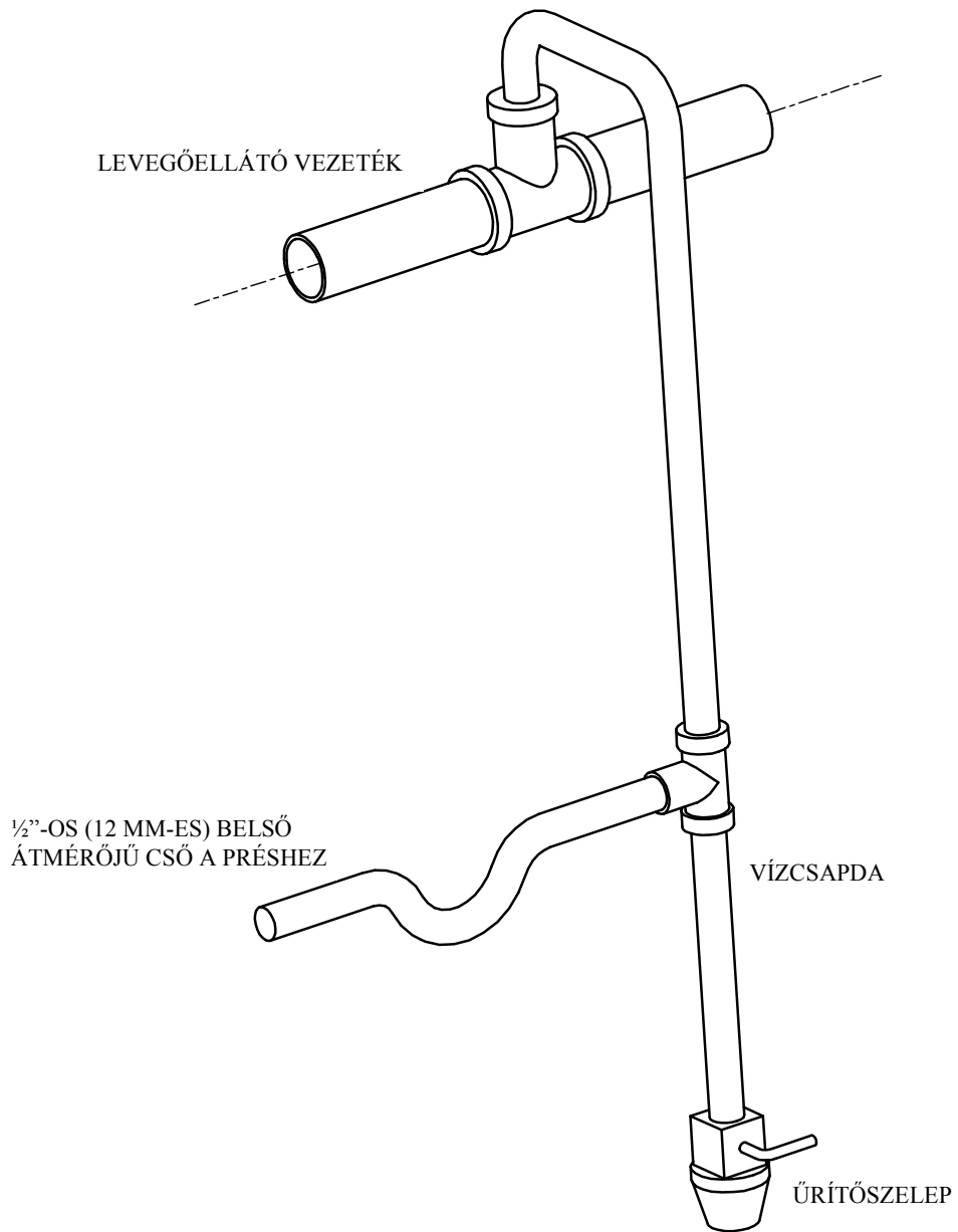
4-2 ÁBRA LEVEGŐELLÁTÁS
