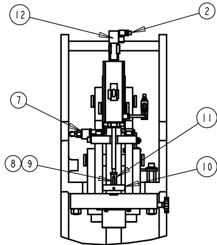
Préskulissza előlnézetben
